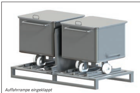
Auffahrrampe eingeklappt
