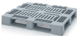
Variante: PAL_H3-5 mit Sicherungsrand 2 Quer- und 3 Längskufen, nicht verschweißt
